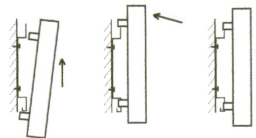
Schemat mocowania na ścianie
