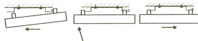
Schemat mocowania na suficie
